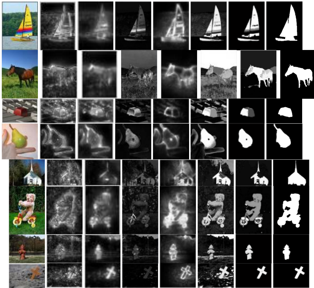
(a)original (b) Itti/Koch (c) GVBS (d) FC (e) CA (f) HC (g) Ours (h) groundtruth
